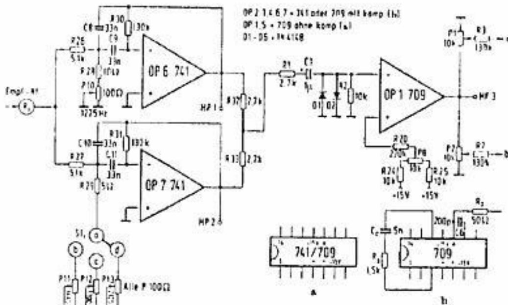
3.11 RTTY-NF-Konverter DJ6 HP 001 Abb. 4 a
