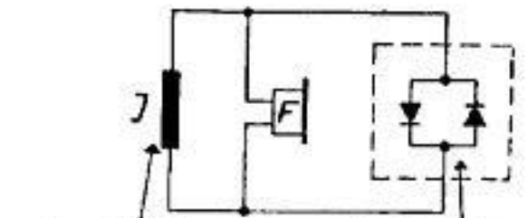
Zweitwicklung der Induktionsspule Gehörschutz-Gleichrichter
