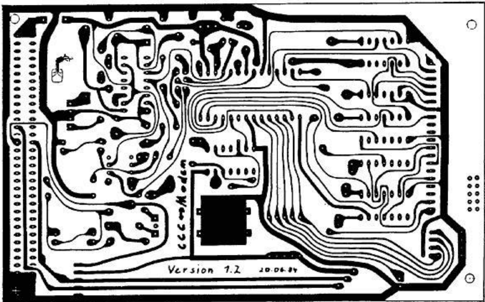
Lötseite
