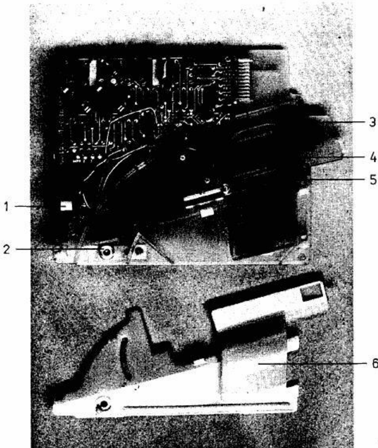
Bild 9: Münzprüfer (Baugruppen 2, 3, 4)
