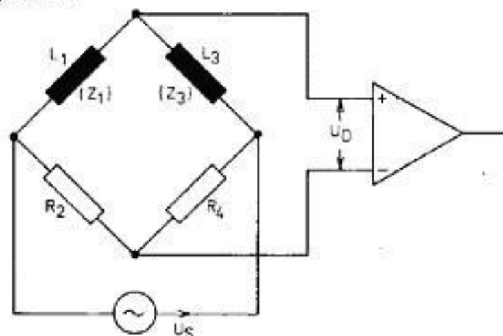
Bild 10: Grundsätzlicher Aufbau der Münzprüferbrücke
